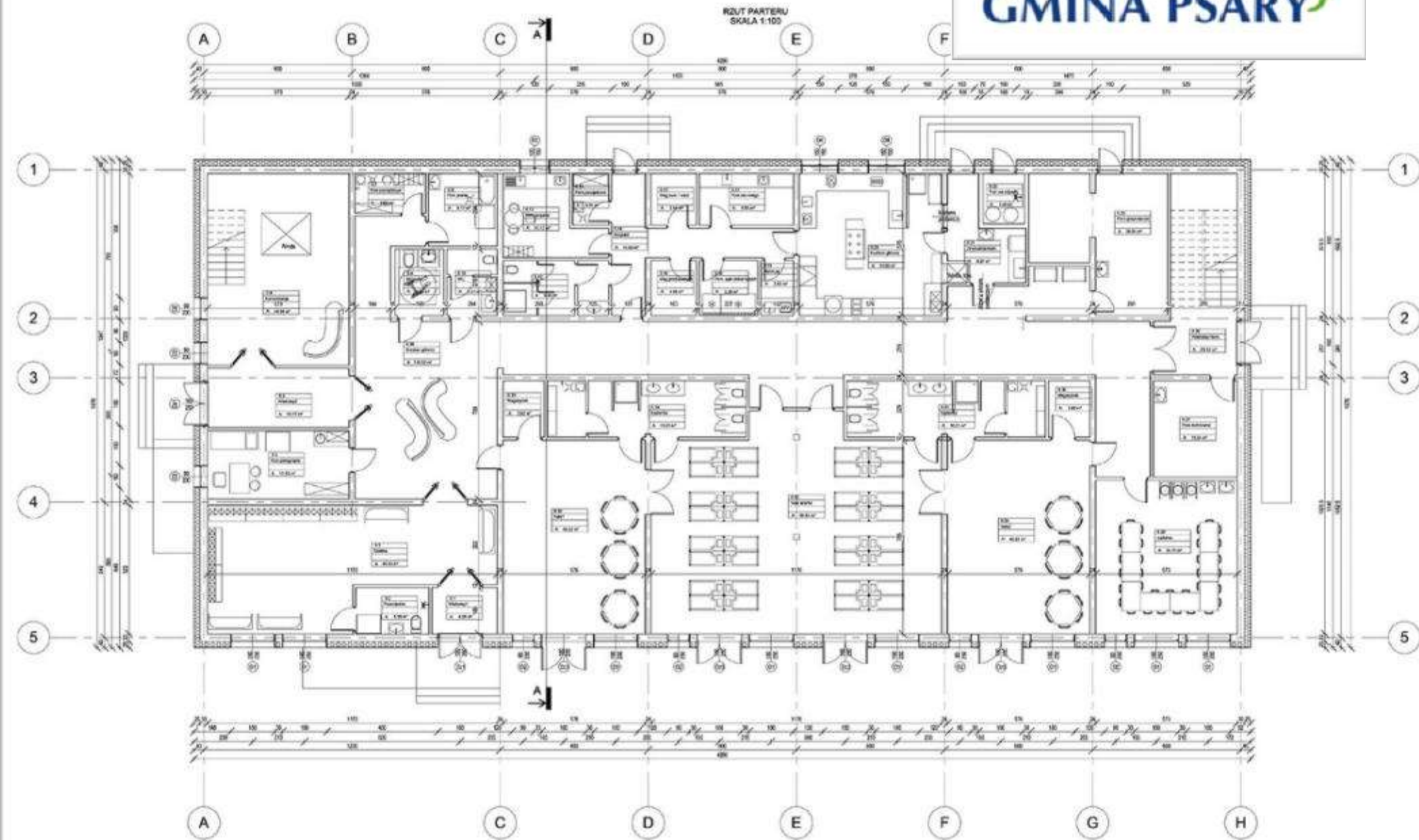
Rzut projektowanego żłobka i przedszkola w Psarach, który będzie budynkiem pasywnym.
