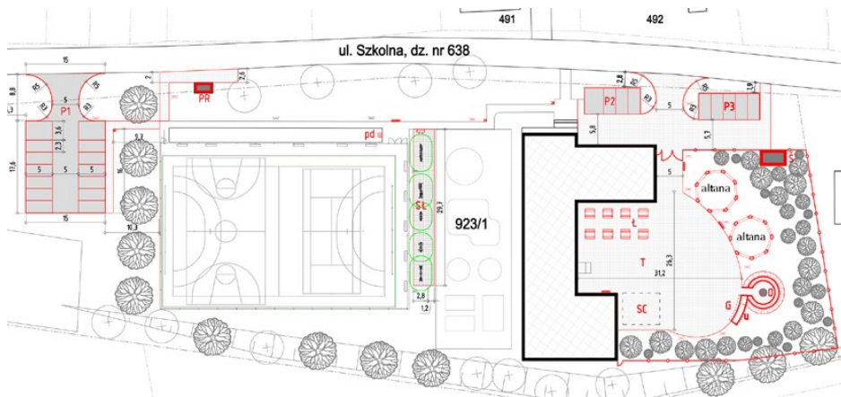
Projekt techniczny zagospodarowania terenu wokół szkoły w Malinowicach
