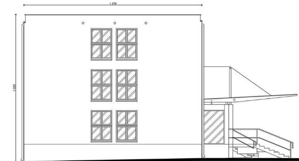
elewacja północna - stan projektowany
