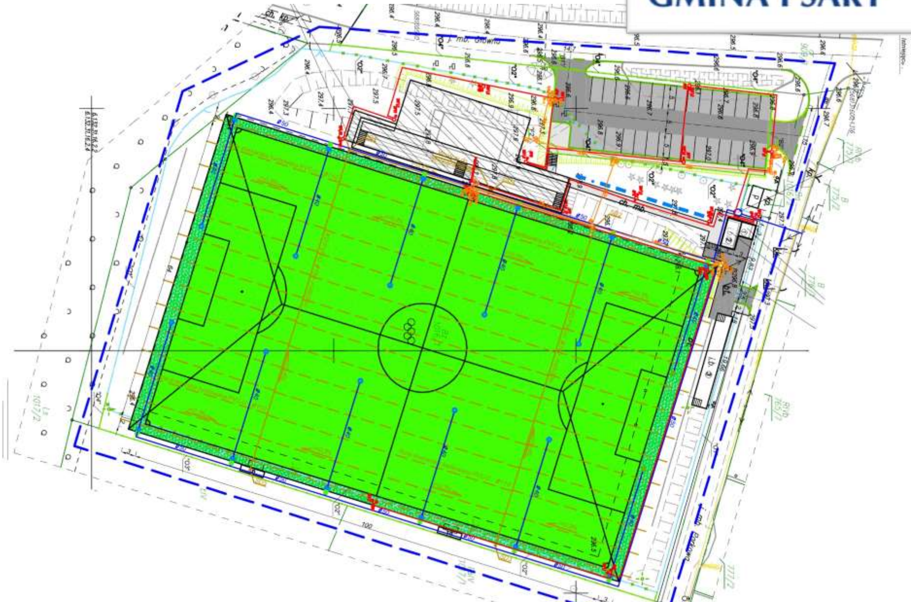
Projekt budowy stadionu Klubu Sportowego Sarnów.
