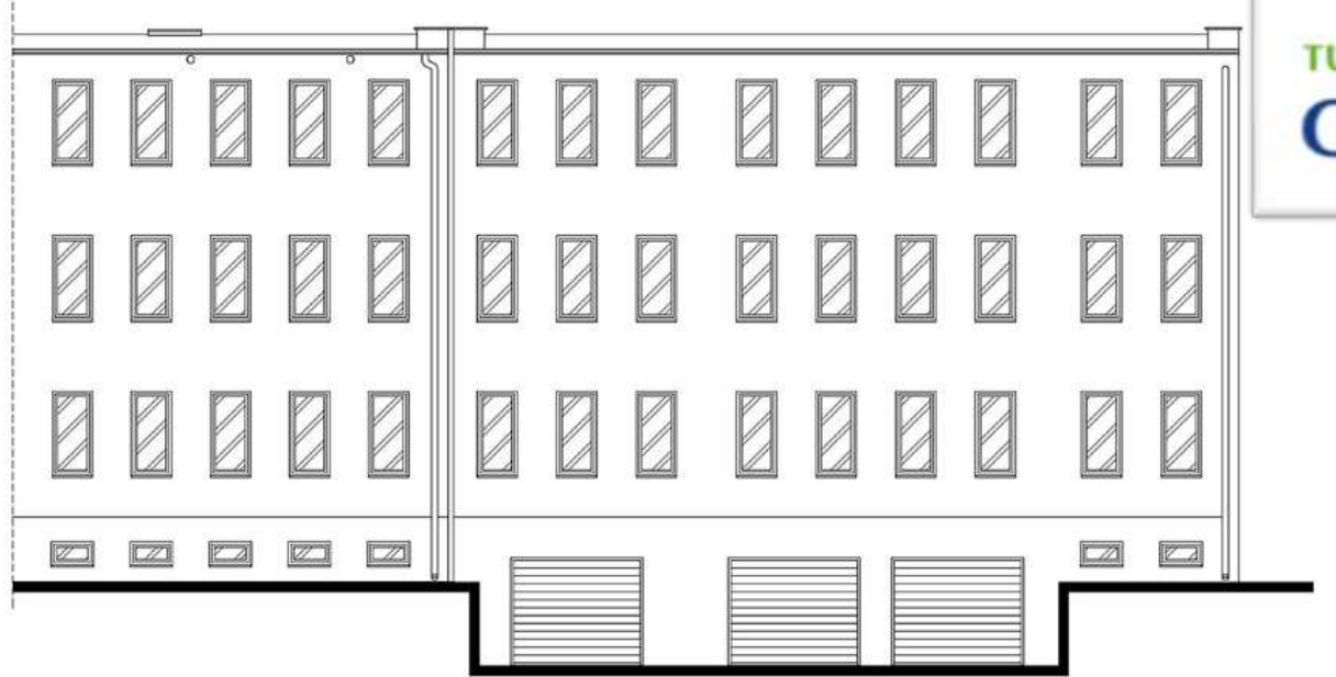
elewacja wschodnia - stan projektowany
